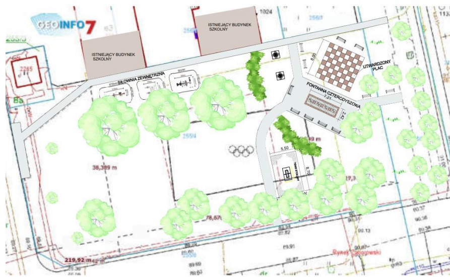
PROJEKT ZAGOSPODAROWANIA TERENU NA RYNKU ZABOROWSKIM
